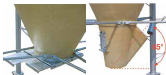
Transparante trechter
